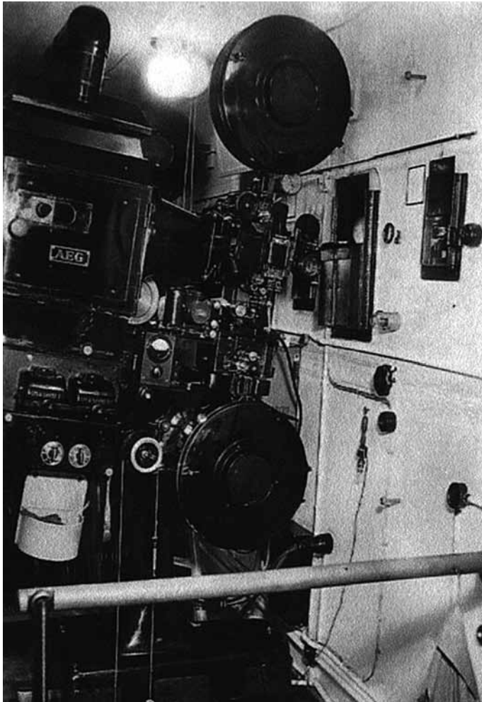
Zu sehen ist eine alte Technik. Ein Filmvorführgerät der Firma AEG. Die Filmbreite betrug 32 mm.
